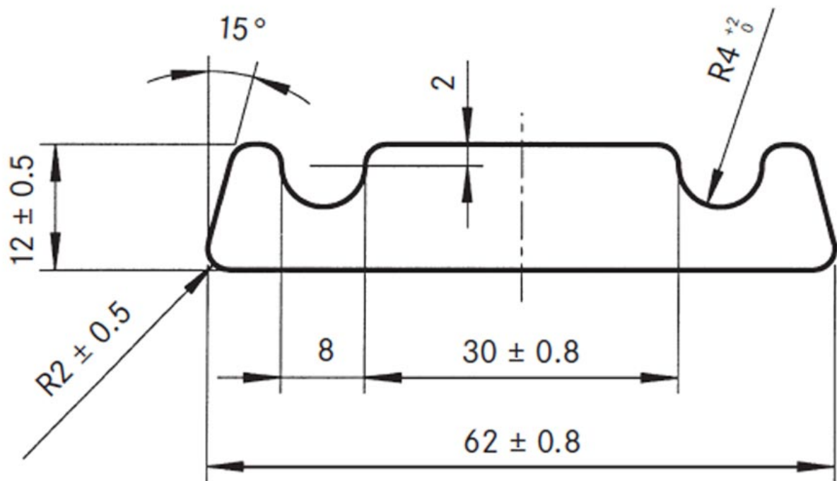
技術図面 RS-1
