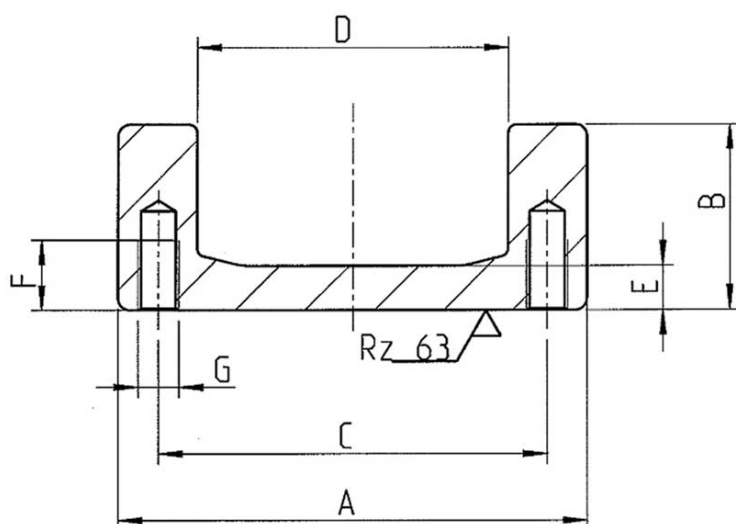
Zeichnungsvorlage für Kundenprofil Drawing for customized profile
