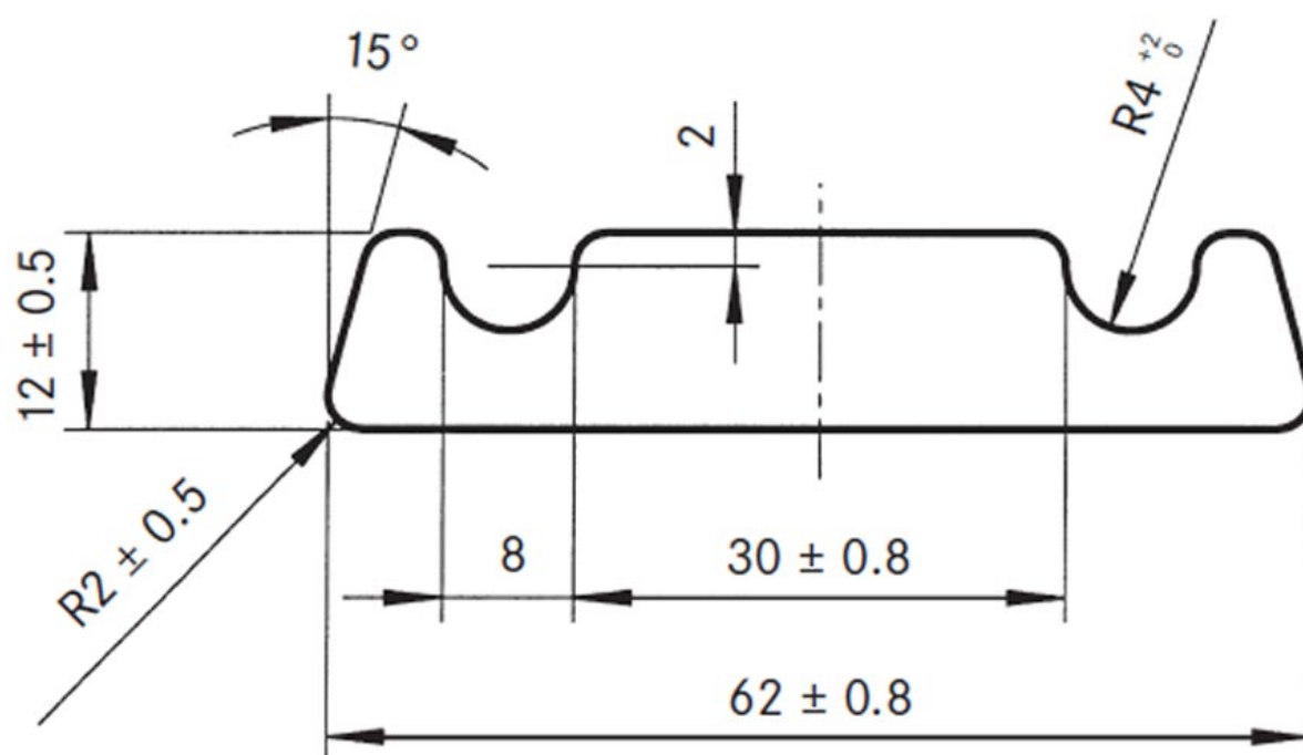
Dibujo técnico RS-1
