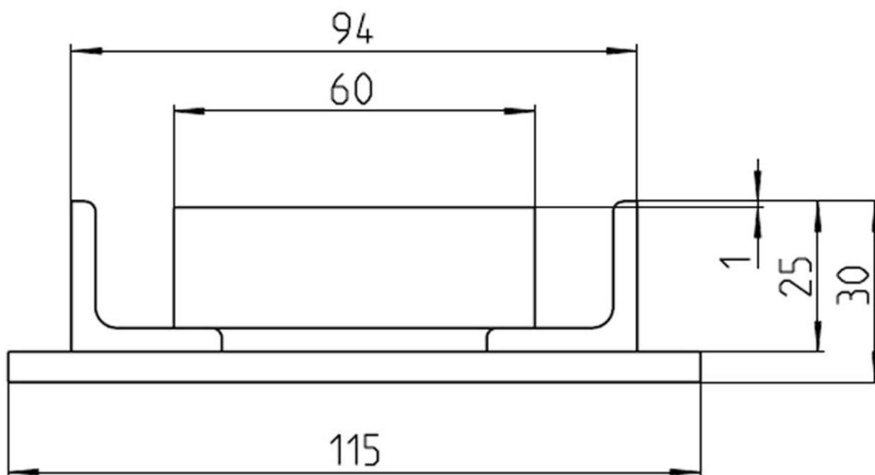
技术图纸 RS-2-FG
